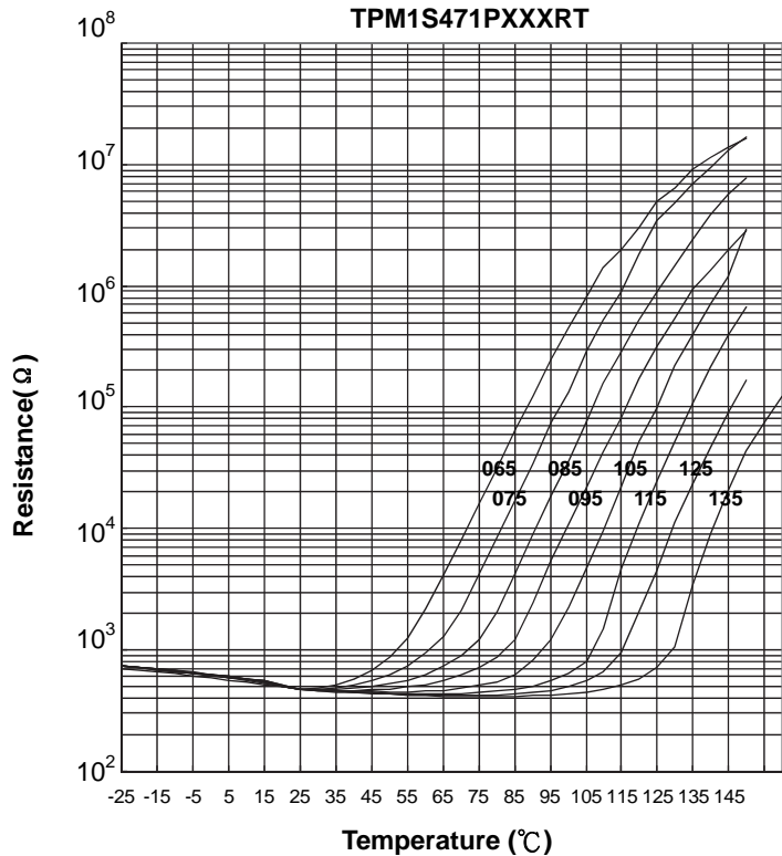
SMD 0603 R25=470Ω
